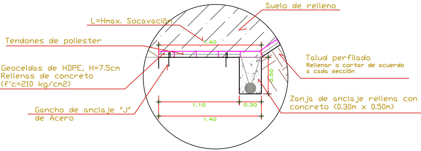
Detalle 3. Anclaje en zanja en fondo de rio y adentramiento final Esc: 1/25
