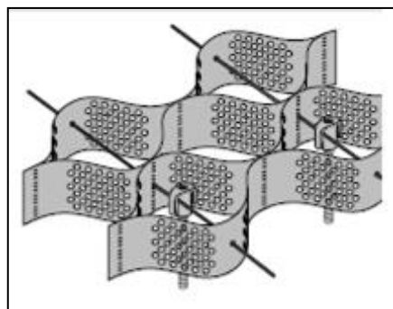
Figura 20: Anclajes internos
