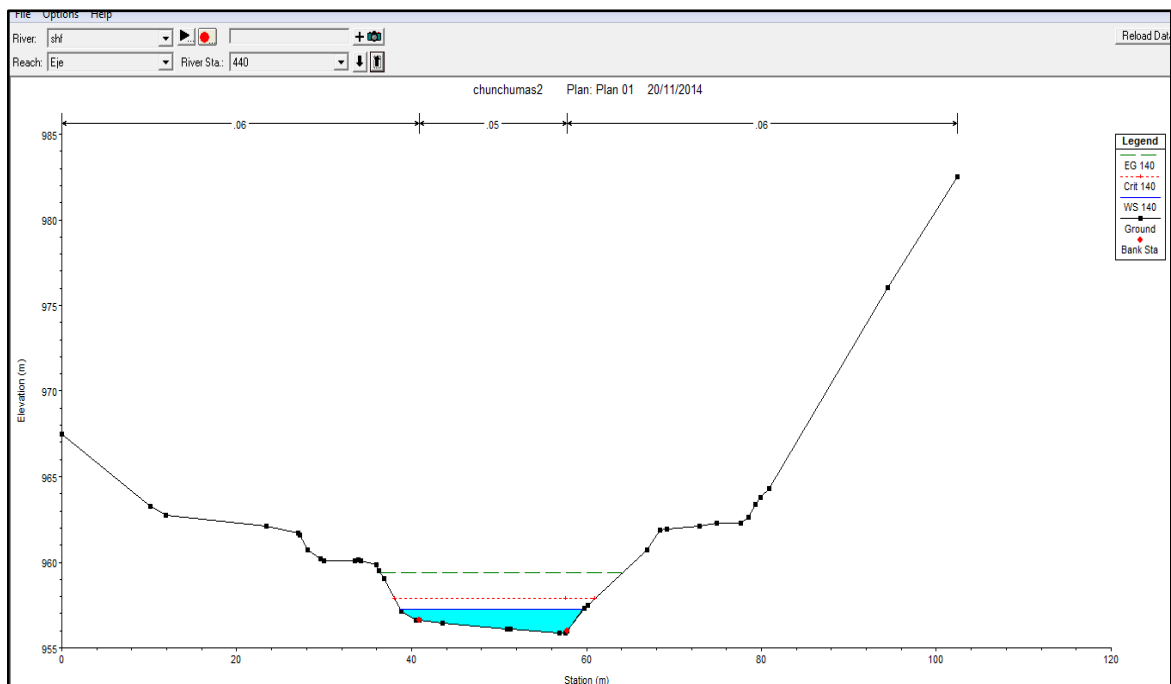
Figura 49: Sección transversal del río sección 0+440
