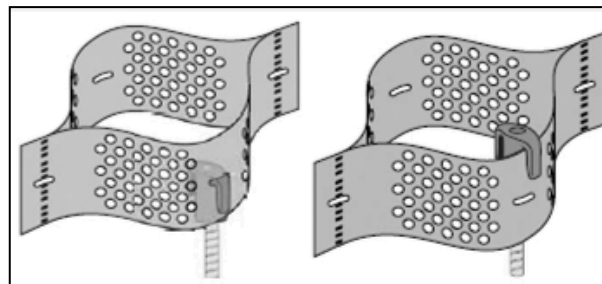
Figura 13: Fijación de borde con ganchos
