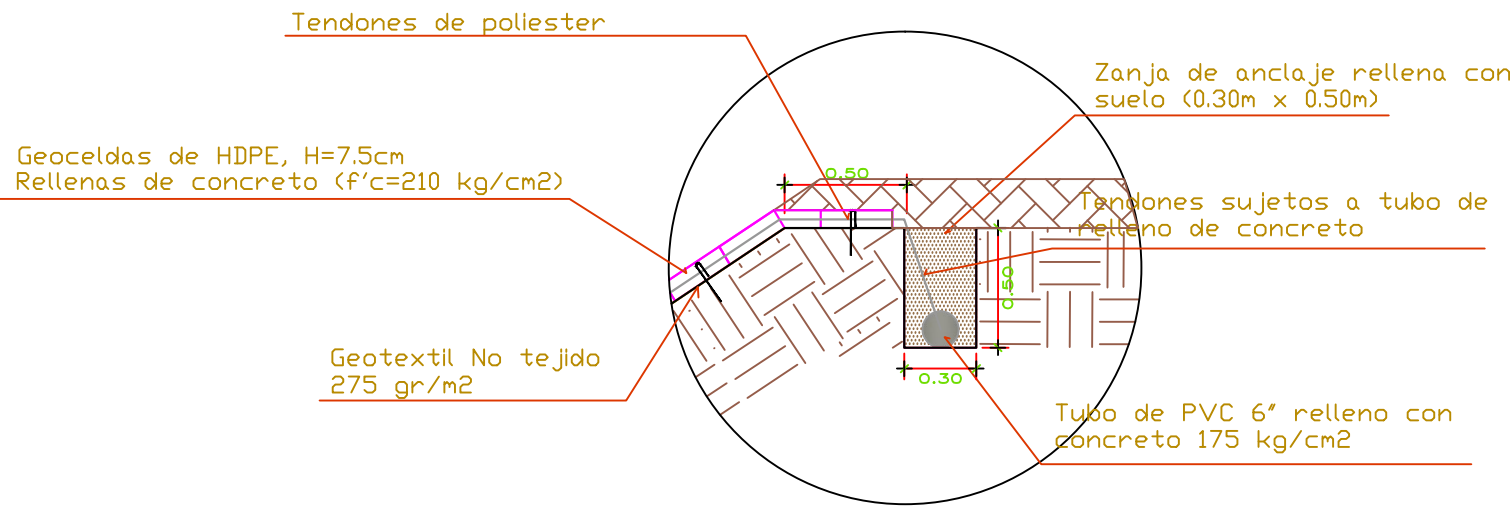
Detalle 1. Zanja de anclaje en corona de talud Esc: 1/25
